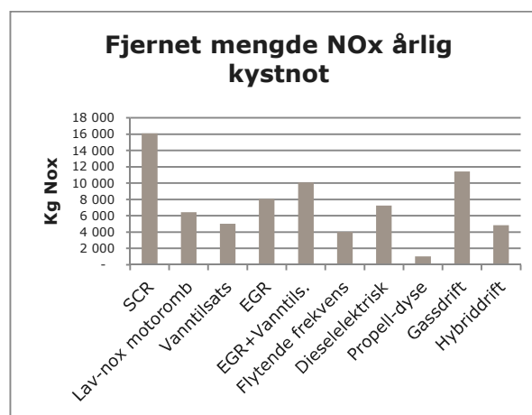
Figur 78: NOx-reduksjon ulike tiltak, kystnot
