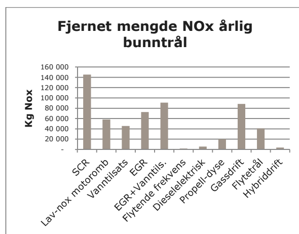
Figur 76: NOx-reduksjon ulike tiltak, bunntål
