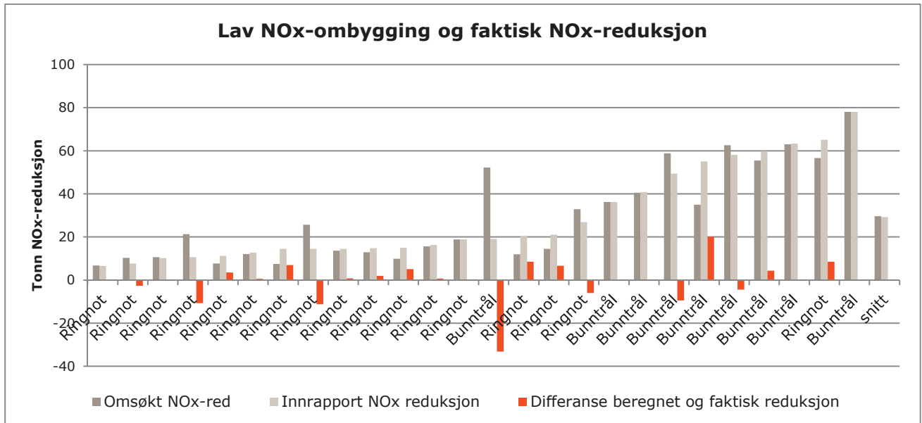
Figur 9: Effekten av tiltaket Lav-NOx-ombygging. Rangering etter mengde faktisk reduksjon.
