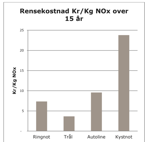
Figur 11: Faktisk renseseffektivitet for Lav-NOx-ombygging. Tallene for autoline og kystnot er beregnede tall basert på en gjennomsnittlig driftsprofil for disse fartøyene.
